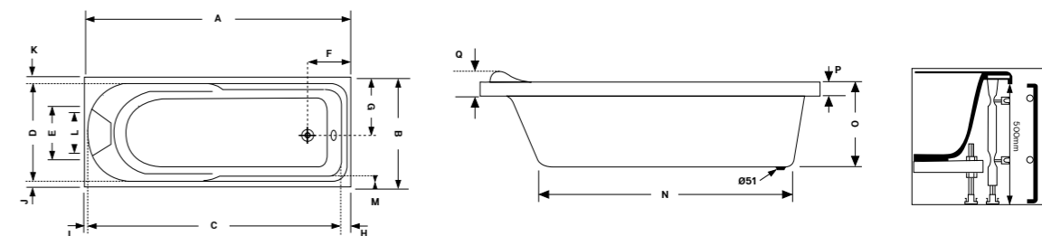
Tolerância +/- 1% Tolerance +/- 1%
