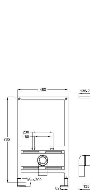
Estrutura para bidé S120/168 Ref.: RESBIDSUSRUB Pack: 11 kg / 0,06 m³
