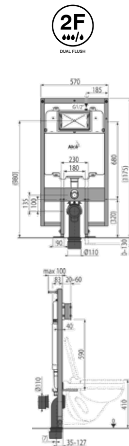
Não inclui placa de accionamento Estrutura para sanitário suspenso e ao chão S200/280 Ref.: RES110ISLM Pack: 17 kg / 0,09 m³
