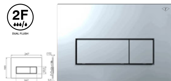
Placa CROMADO S36/50.4 Ref.: RPLM571CRM Pack: 0,34 kg / 0,0016 m³
