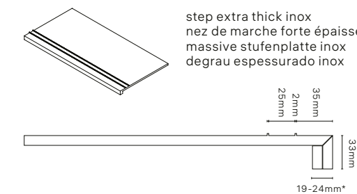
step extra thick nez de marche forte épaisseur massive stufenplatte degrau espessurado
