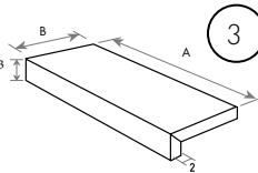
PELDAÑO GRD 20MM RECTO GRD 20 MM STRAIGHT STEP
